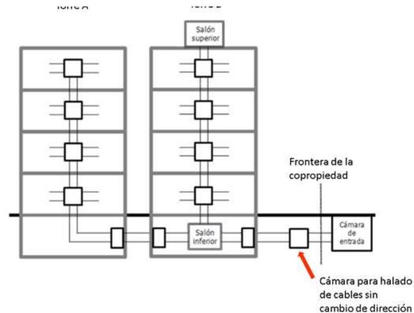
Ilustración 1. Ejemplo de copropiedades de dos torres compartiendo un SETI y un SETS. Fuente: Propia.
