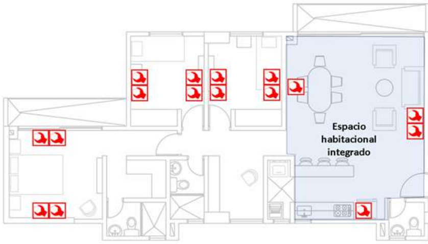
Ilustración 23. ubicación de las cajas de toma de usuario en una vivienda de más de 280 SMMLV con el espacio habitacional de la cocina integrado con espacios de otros usos. Fuente: Propia.
