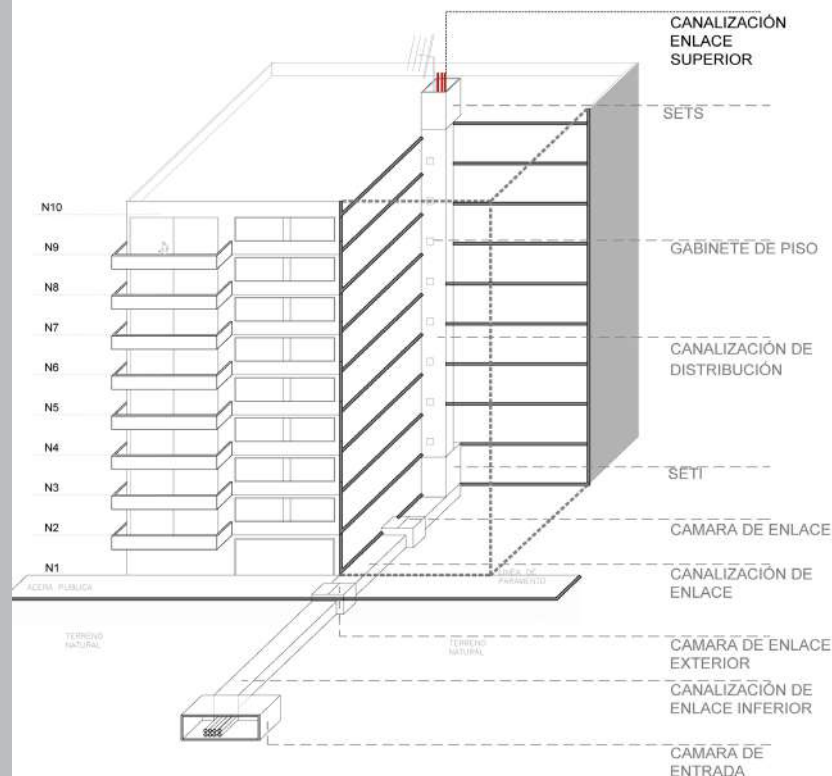
Ilustración 25. ubicación de los elementos de captación, cabecera y difusión.
