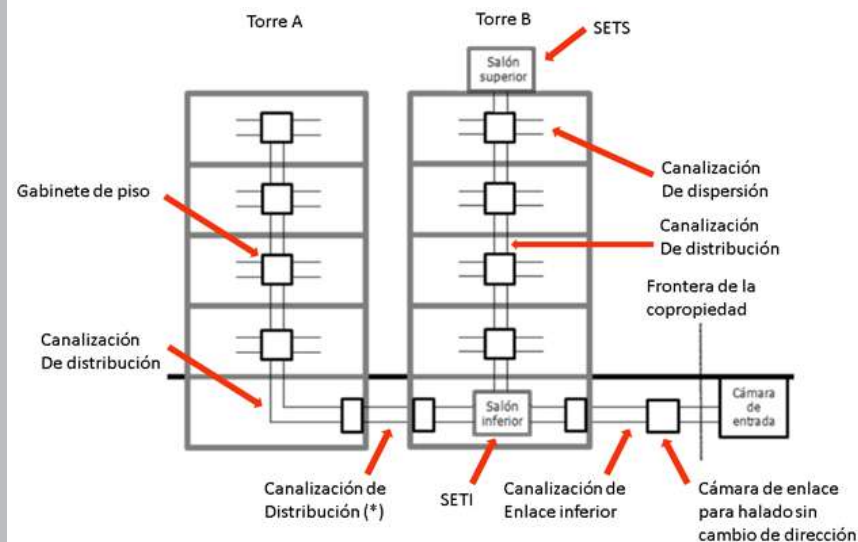
Ilustración 2. Identificación de los componentes de la infraestructura soporte en el ejemplo de copropiedades de dos torres compartiendo un SETI y un SETS. Fuente: Propia.
